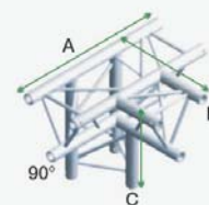
Angle X30 - Cross UP/Down - 6 way FT30-022 Réf: LS0215022
